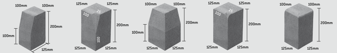
KL HB or BN 100 x 127 x 200mm KL HB Internal Corner KL HB External Corner KL BN Internal Corner KL BN External Corner
